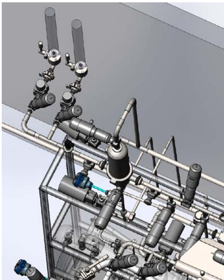
3D-модель обвязки
