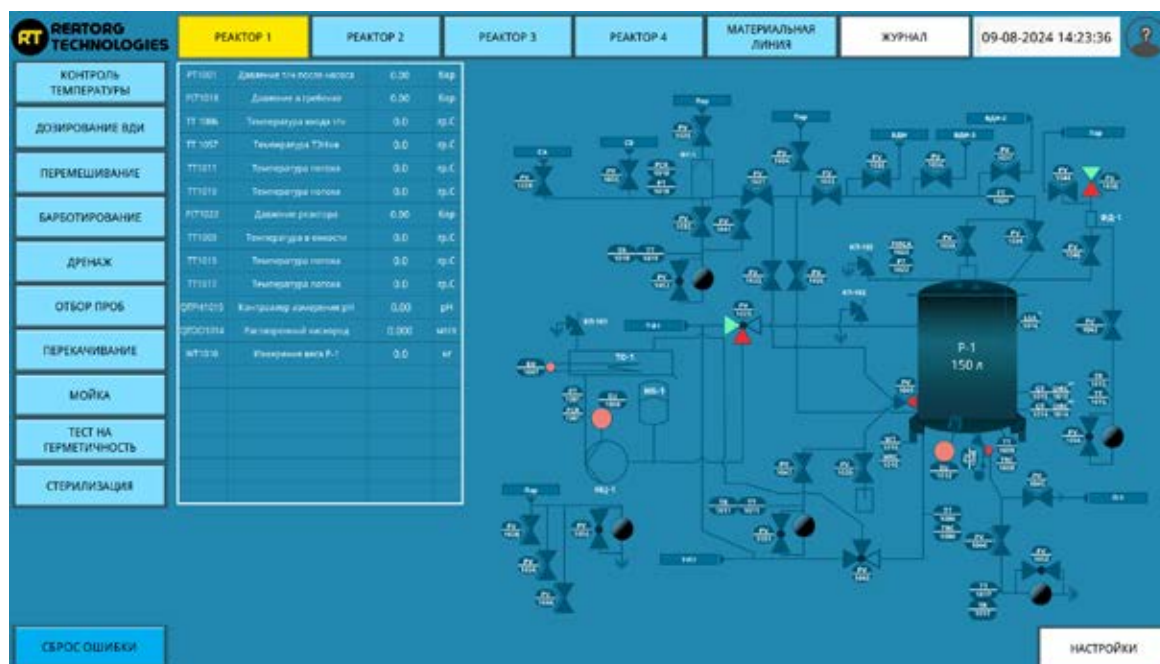
Панель управления
