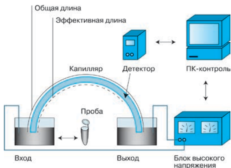
Принципиальная схема СКЭ
